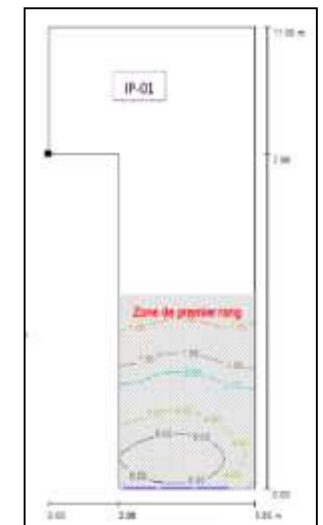
Résultats de calcul de FLJ
